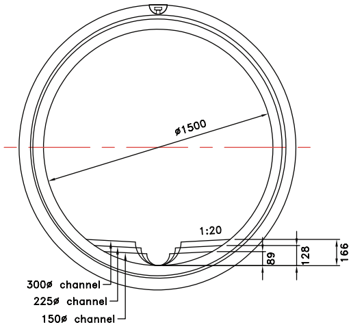
End elevation
